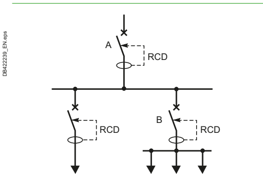
Fig. F15 Distribution circuits
