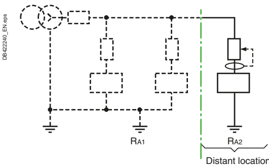
Fig. F16 Separate earth electrode
