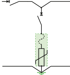
Fig. J34 SCPD "in parallel"
