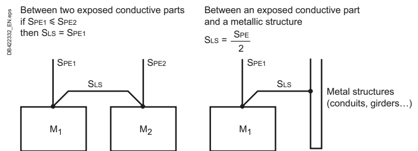
Fig. G63 Supplementary equipotential conductors
