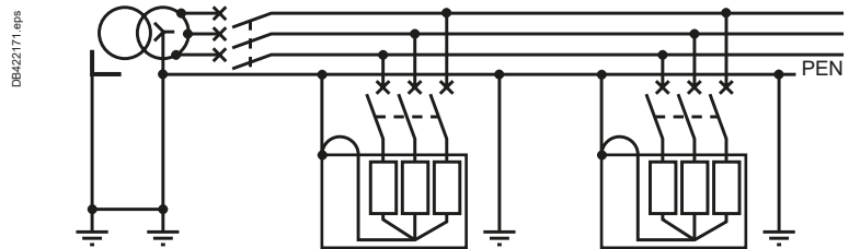
Fig. E13 TN-C system
