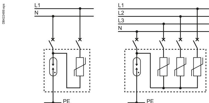
Fig. J29 1P + N, 3P + N SPDs
