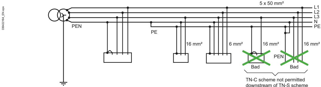
Fig. E6 TN-C-S system
