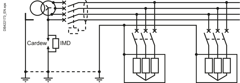
Fig. E15 IT system
